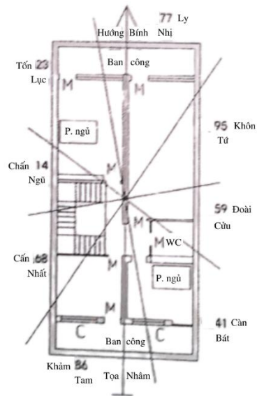
(Mặt bằng phong thủy tầng 2)
